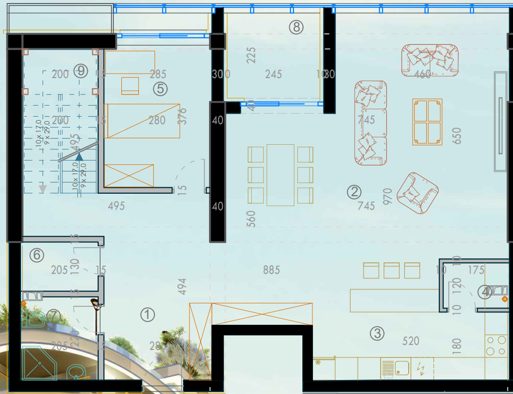
TLOCRT STANA IX ETAŽA 1:100
