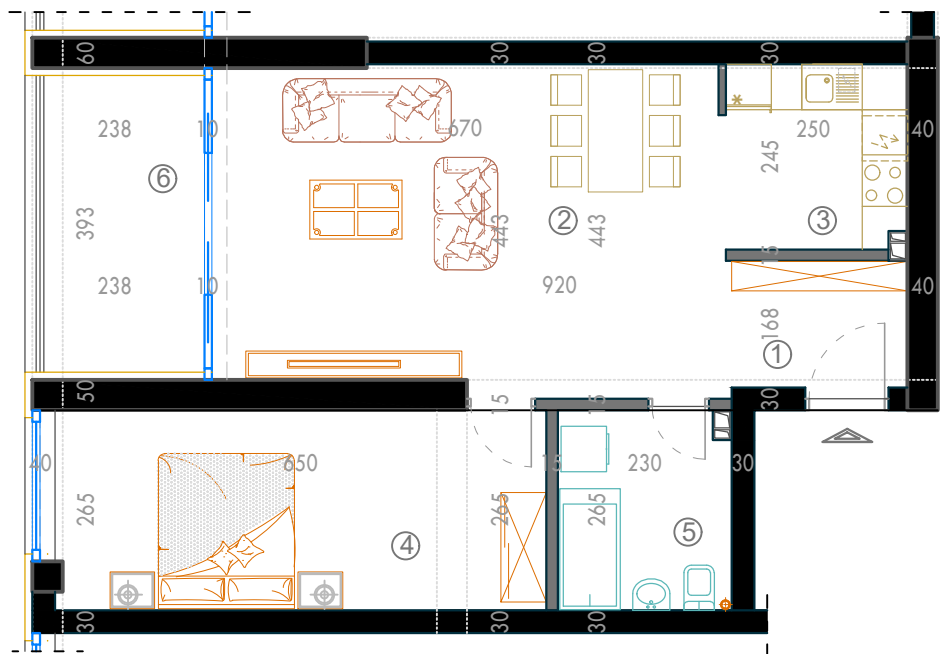
TLOCRT STANA 1:100
