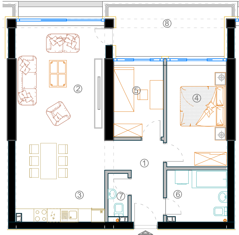
TLOCRT STANA 1:100
