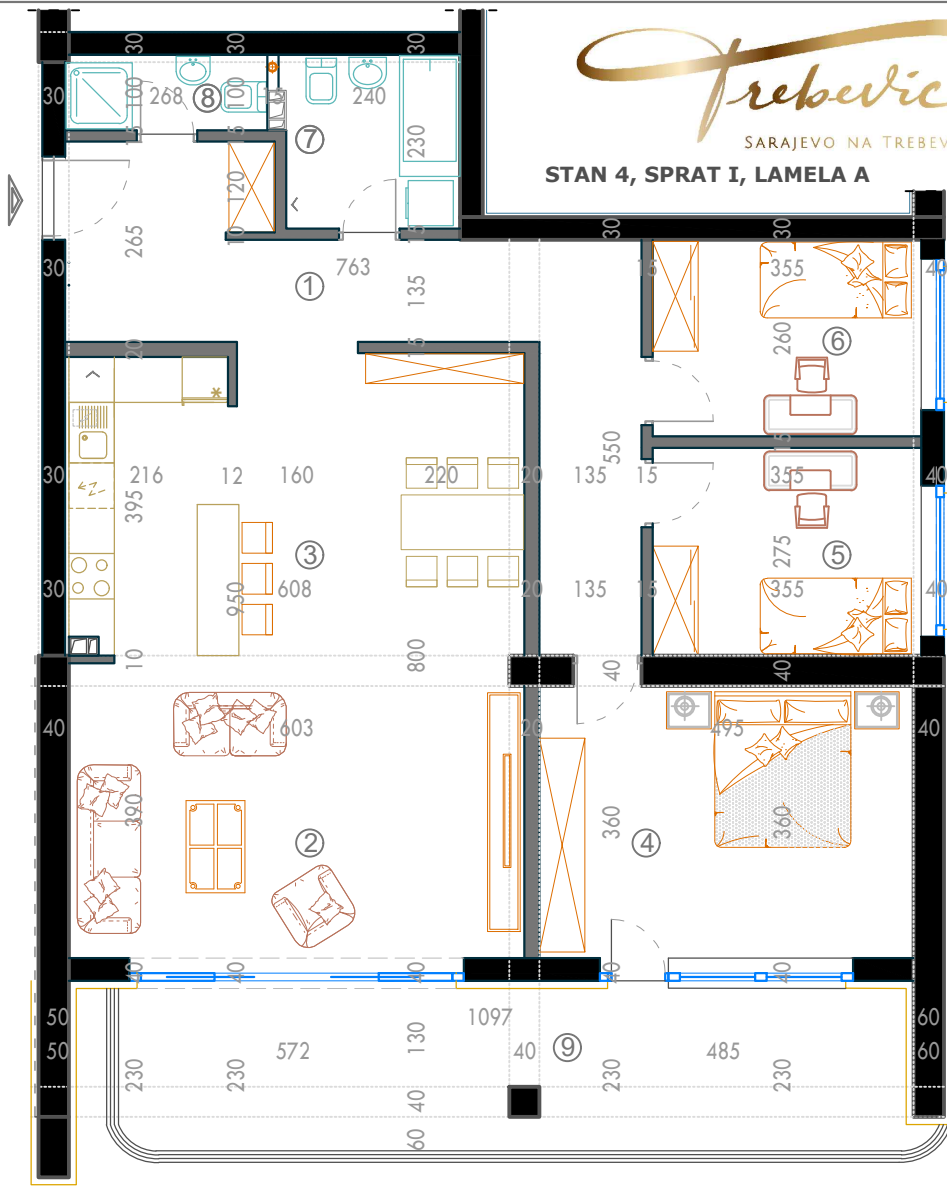
TLOCRT STANA 1:100
