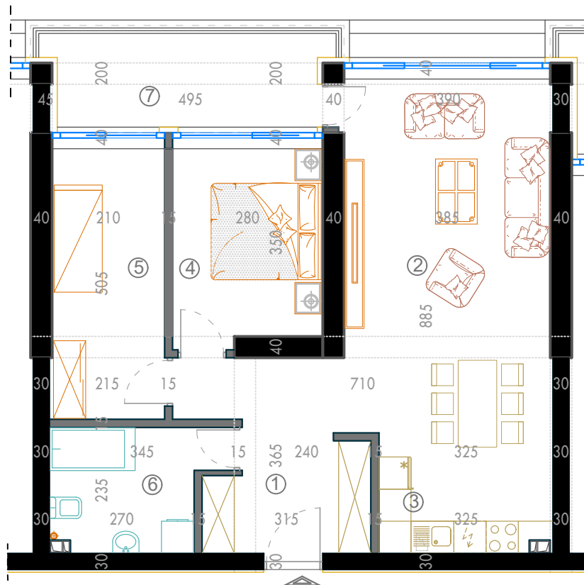
TLOCRT STANA 1:100
