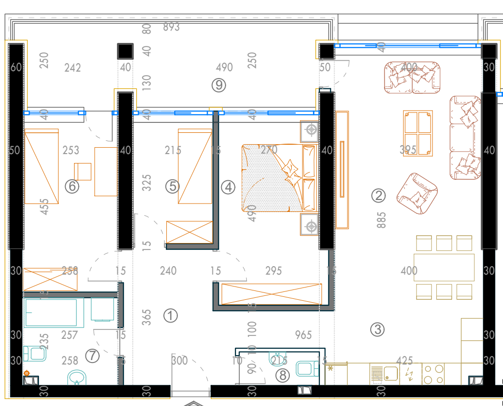
TLOCRT STANA 1:100
