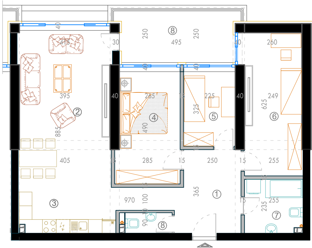
TLOCRT STANA 1:100
