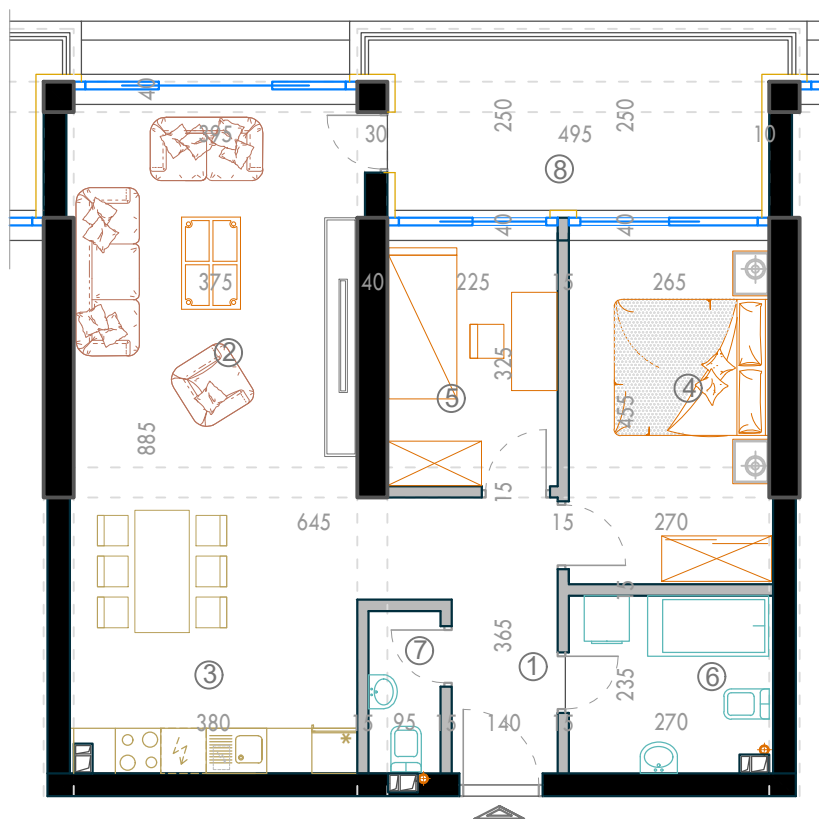
TLOCRT STANA 1:100
