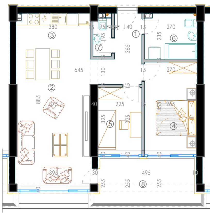
TLOCRT STANA 1:100
