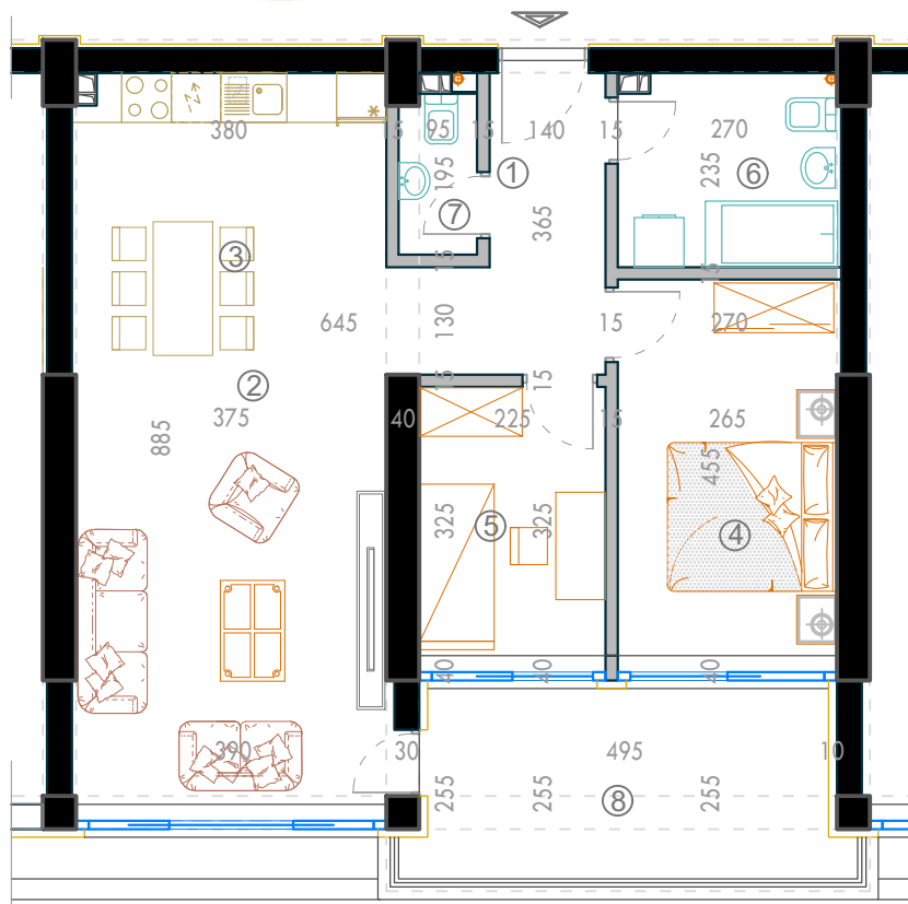
TLOCRT STANA 1:100
