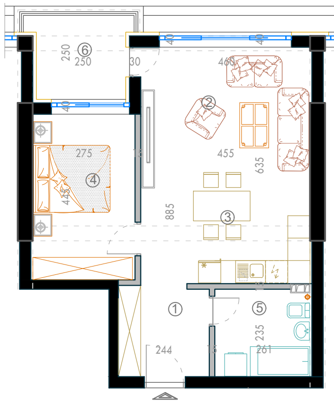
TLOCRT STANA 1:100
