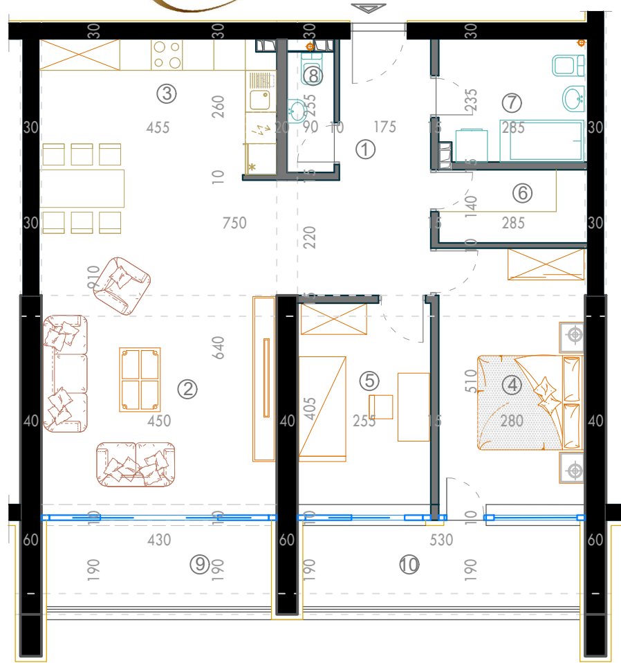
TLOCRT STANA 1:100
