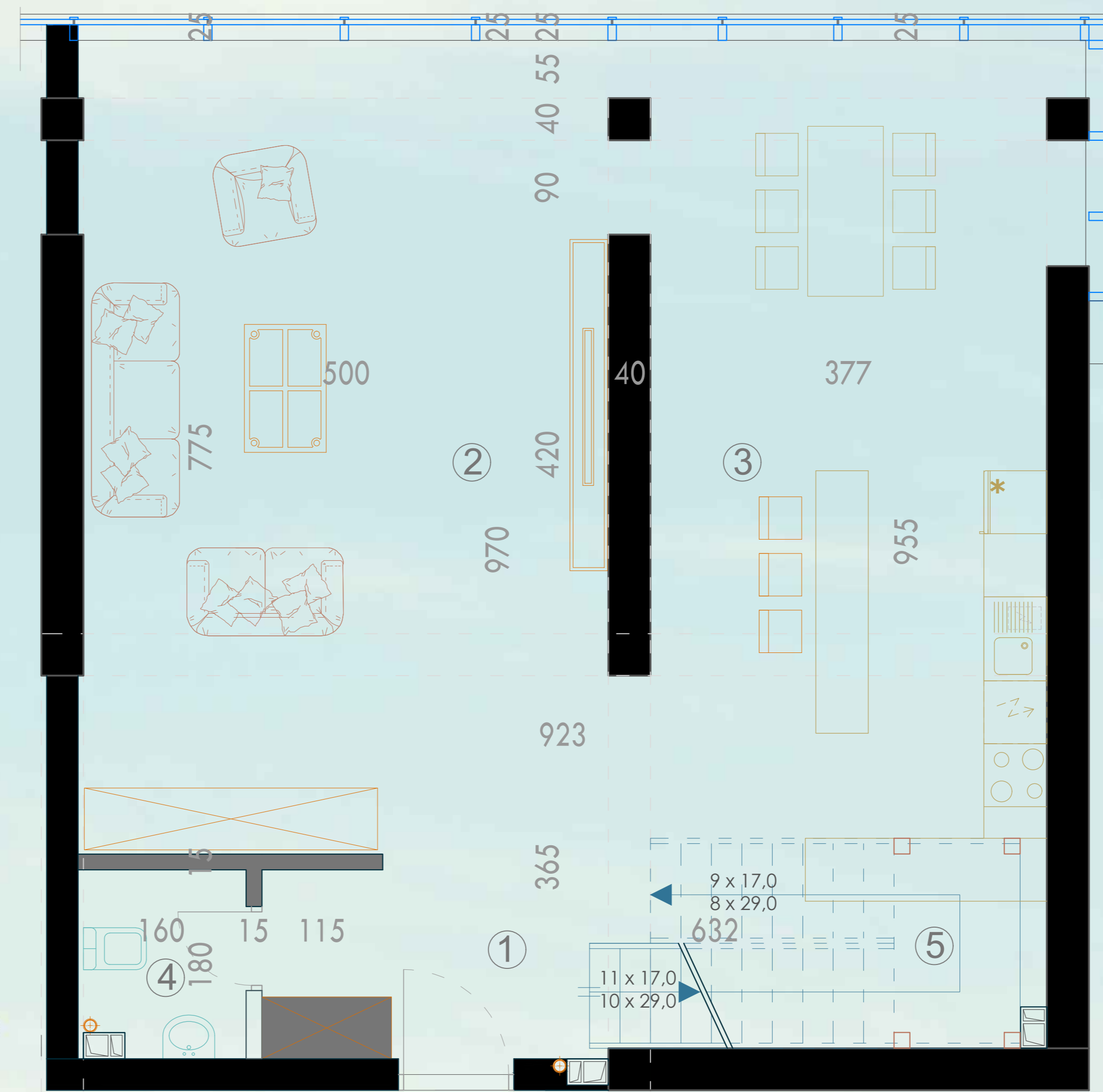
TLOCRT STANA XI ETAŽA 1:100 S15 158,60m²
