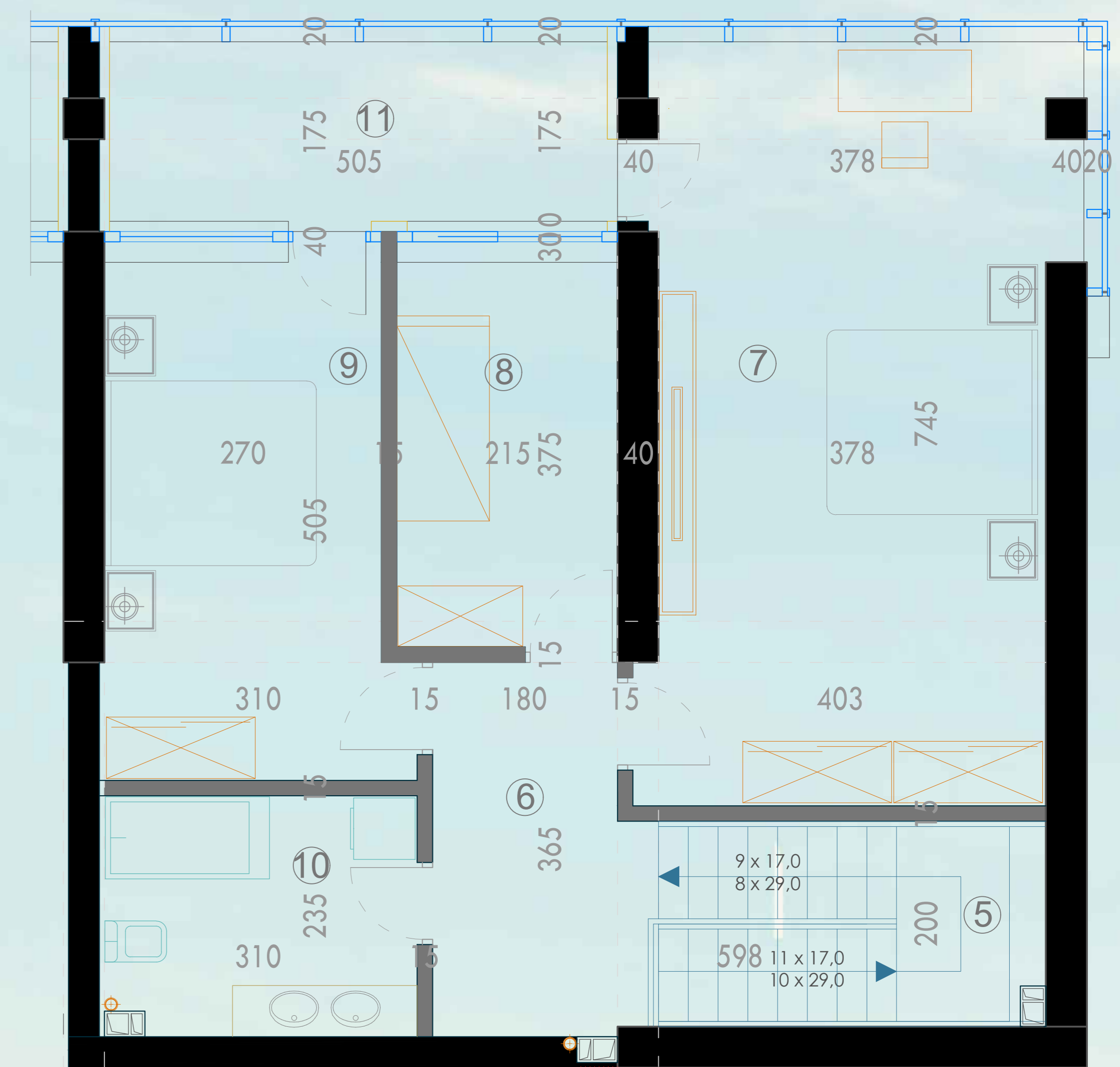
TLOCRT STANA XII ETAŽA 1:100
