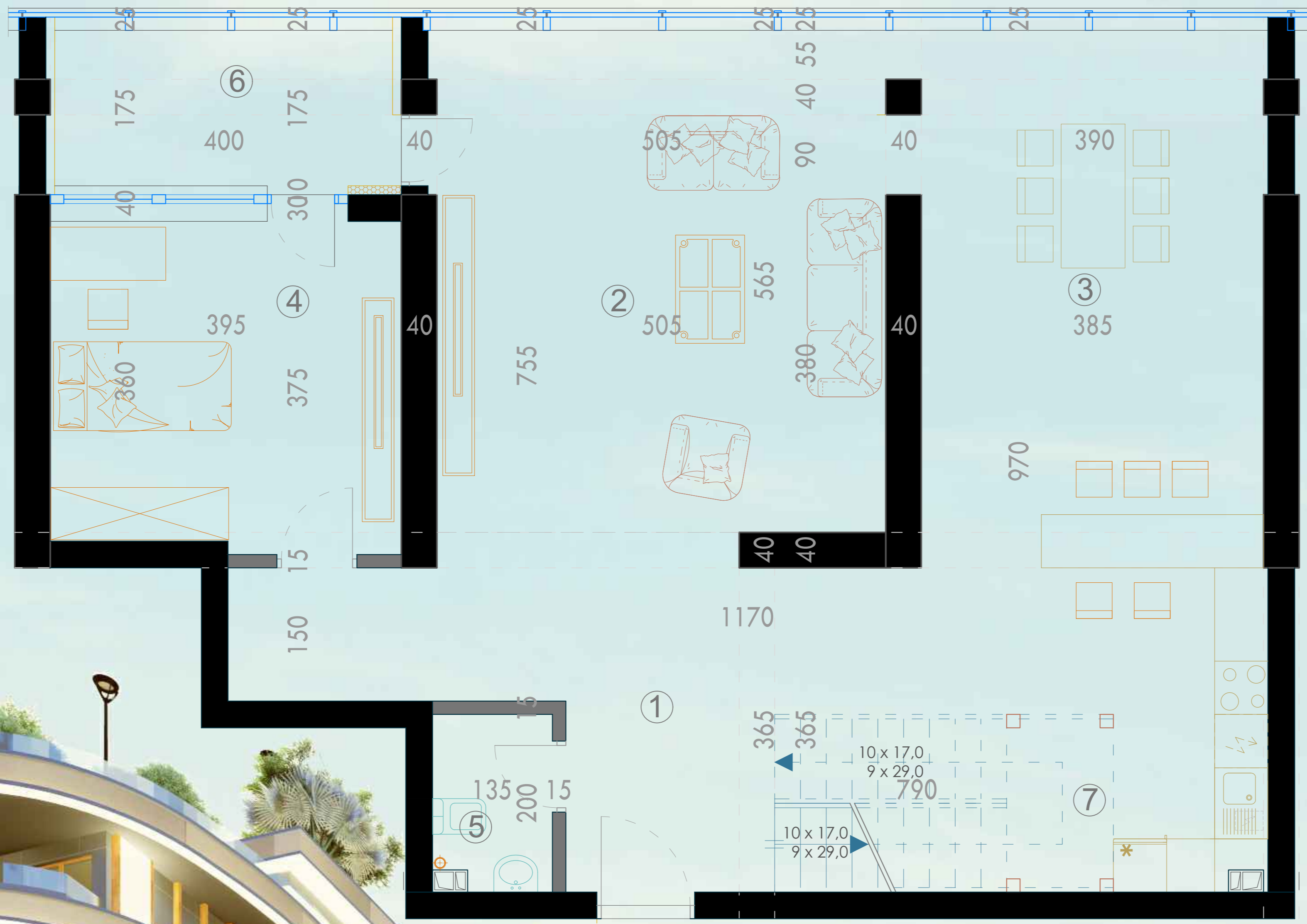
TLOCRT STANA XI ETAŽA 1:100
