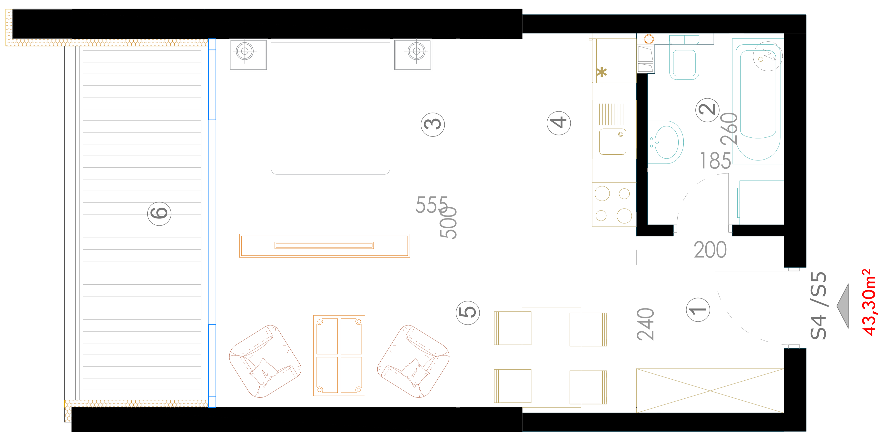
TLOCRT STANA 1:100
